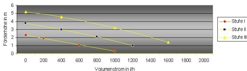
Restförderhöhe UNIA-Mischheizkreis
